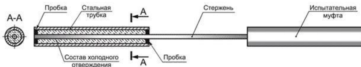
Рисунок В.1 – Вид типового опытного образца
