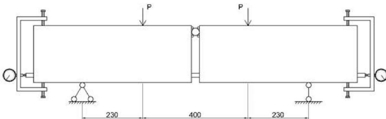
Рисунок Е.4 - Схема испытания образца изгибом балки
