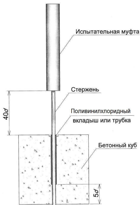
Рисунок Е.1 - Схема установки АКП в бетон куба
