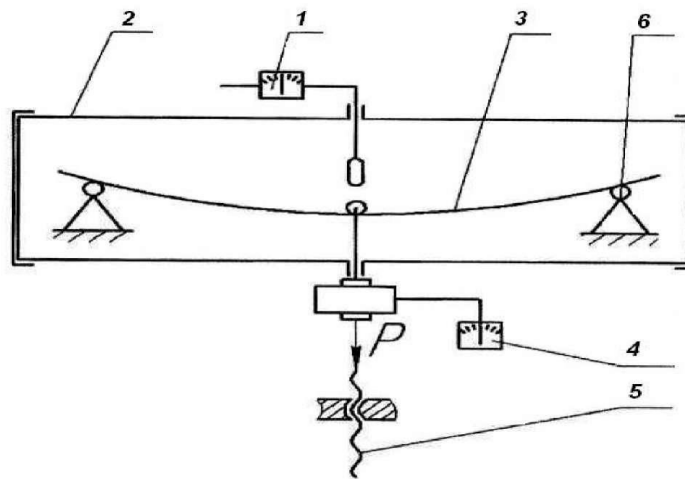
1 - датчик измерения температуры; 2 - нагревательная камера; 3 - образец; 4 - датчик измерения силы; 5 - нагружающий механизм; 6 - опора Рисунок И.2 - Схема испытания образца при определении температуры начала размягчения опытного образца
