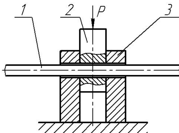
Рисунок Д.1 – Приспособление для испытания образцов на поперечный срез
